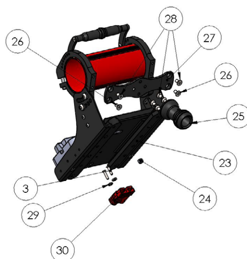
Vue éclatée du sous-ensemble central et électronique
